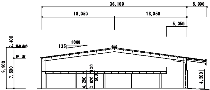
倉庫断面図
