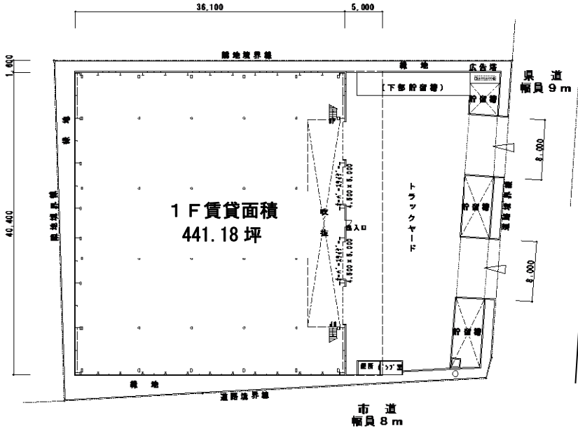
配置図
