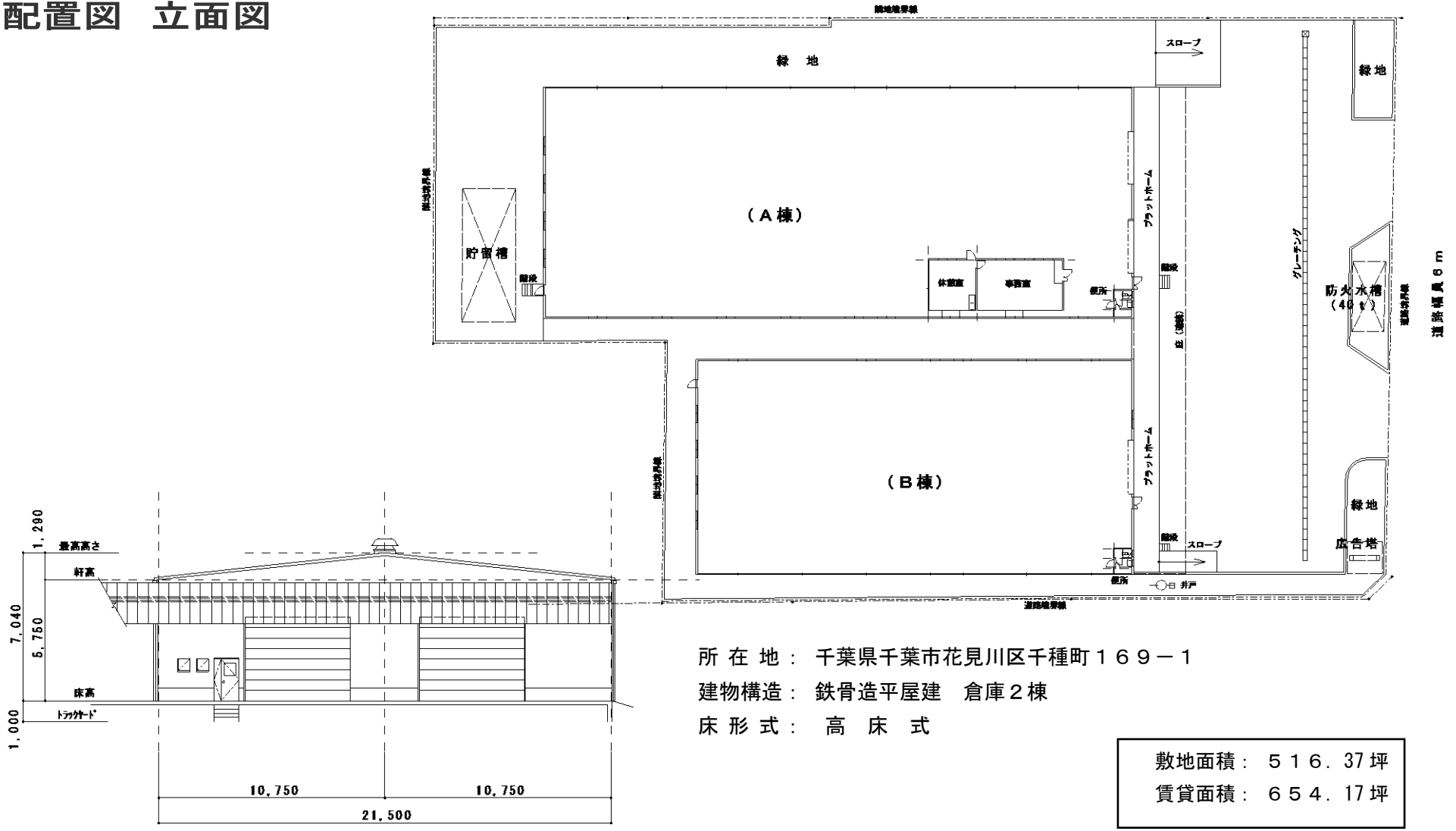
A棟東側立面図
